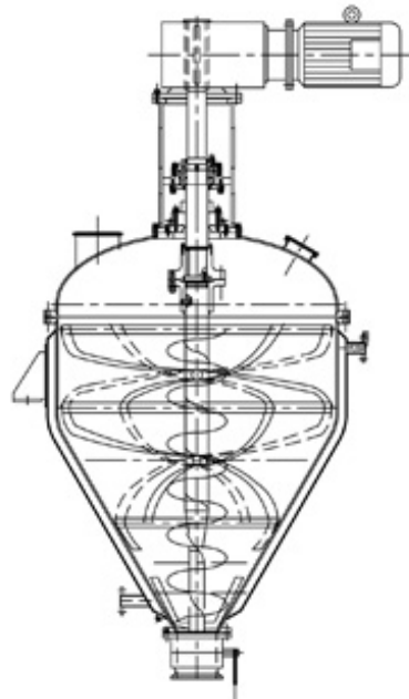
直筒锥底结构
