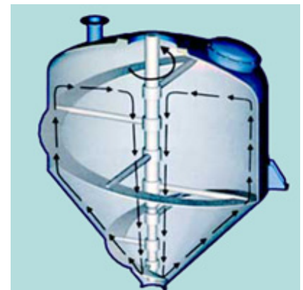
立式螺带运行原理图
